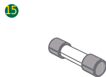
⑮ Alarm relay HRC 6.3A fuse / 5 x 20mm Fusible HRC 6,3A installé en usine Part No. / Référence 3004180
