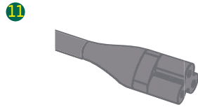
⑪ Power cable / Câble d'alimentation SVT 18AWG*3C Cable +H05VV-F 3G 0.75mm 2 Part No. / Référence 3004139
